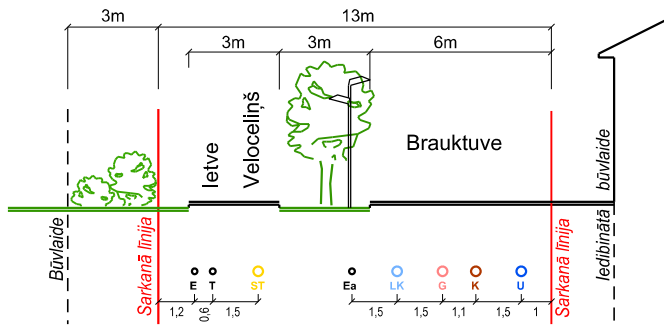
PRIEKŠLIKUMS IELAS PROFILAM A - A
