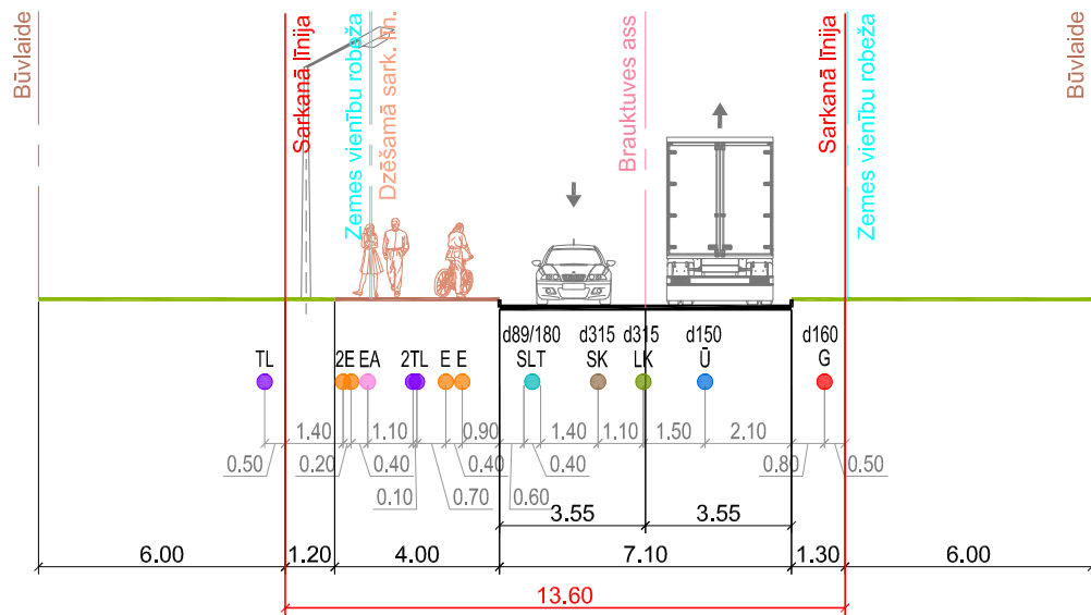
Šķēršprofils 1-1 Krūmu iela
