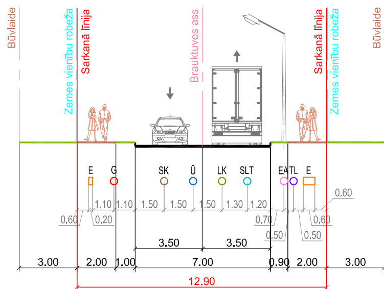
Šķēršprofils 2-2, var.2 Krūmu iela (persp. Mazā Krūmu iela)
