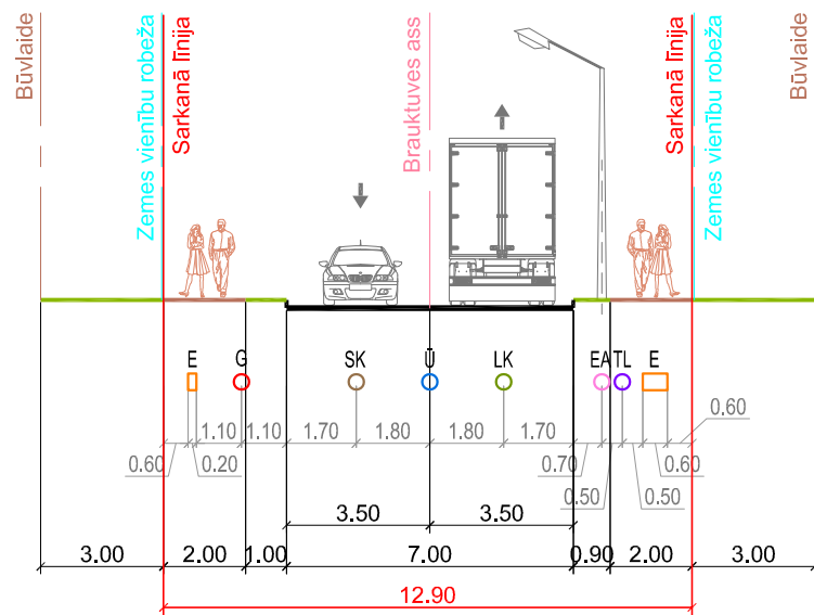
Šķēršprofils 2-2, var.1 Krūmu iela (persp. Mazā Krūmu iela)
