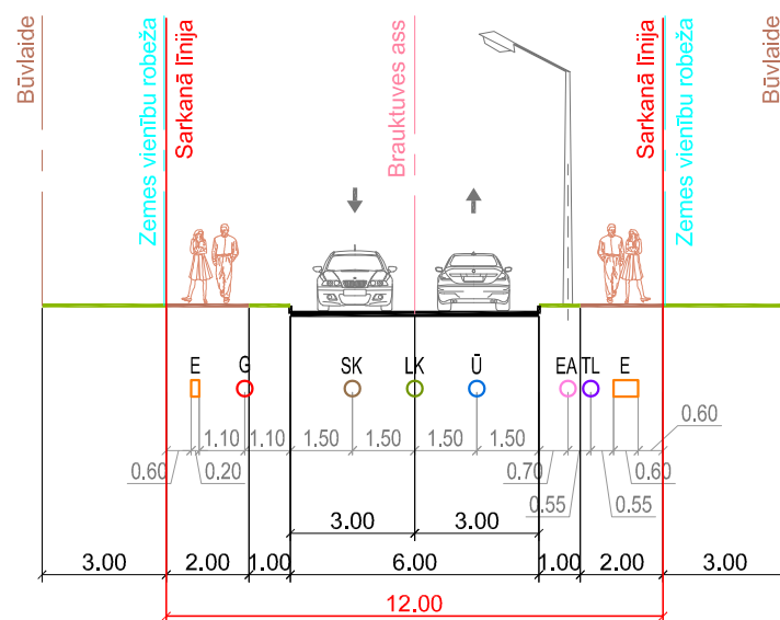
Šķēršprofils 5-5 Jūrkalnes iela
