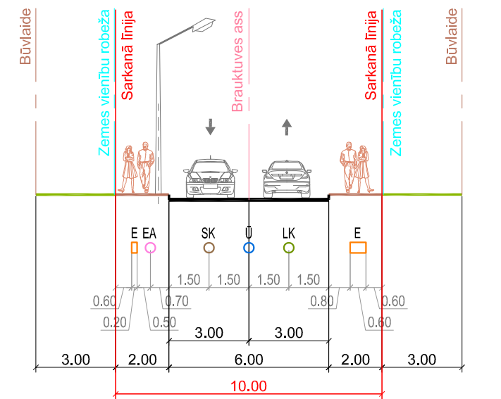
Šķēršprofils 7-7 Mazirbes iela
