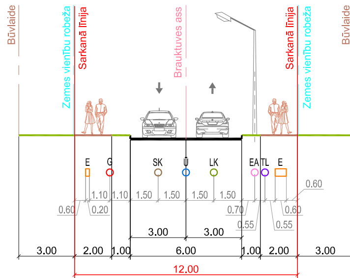
Šķēršprofils 3-3 Kolkas iela
