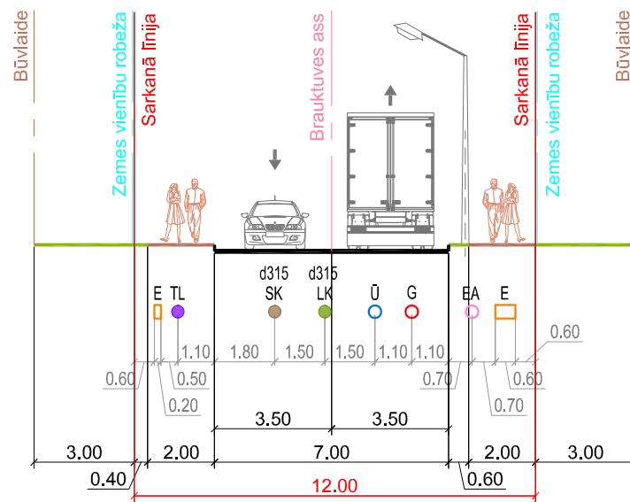
Šķēršprofils 4-4 Jūrkalnes iela
