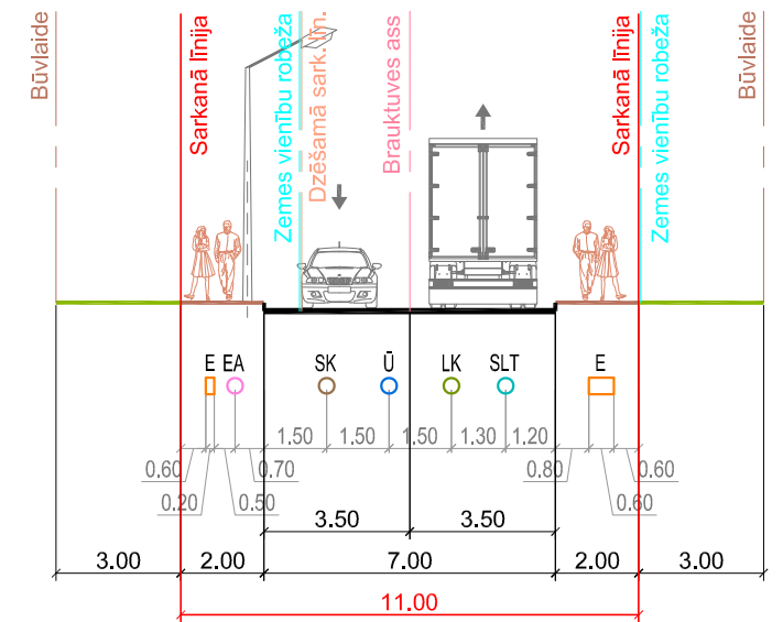
Šķēršprofils 6-6 Mazirbes iela
